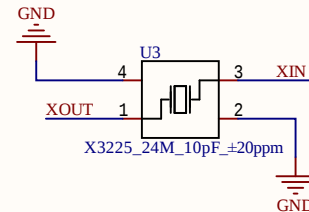
晶振
