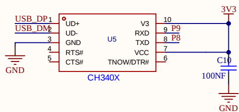
USB转串口芯片
