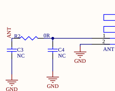
射频部分
