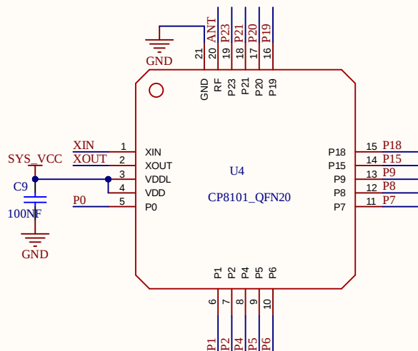
CP8101
