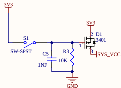
硬件复位电路/电源控制
