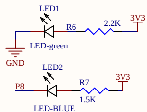
指示灯部分
